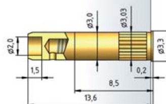
H 5110/GR
