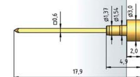
IK 6030.00
