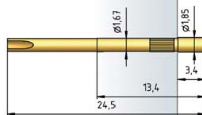
H 1015/GR-L
