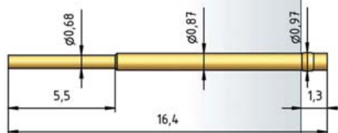
H 1007 C
