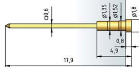
IK 6010.00
