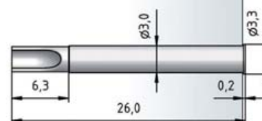
H 2050 L
