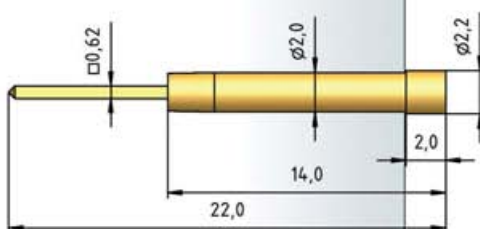
IK 6020.00
