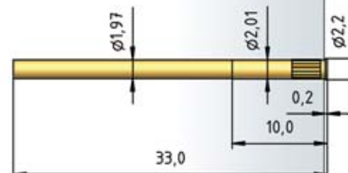
H 1021/GR-C
